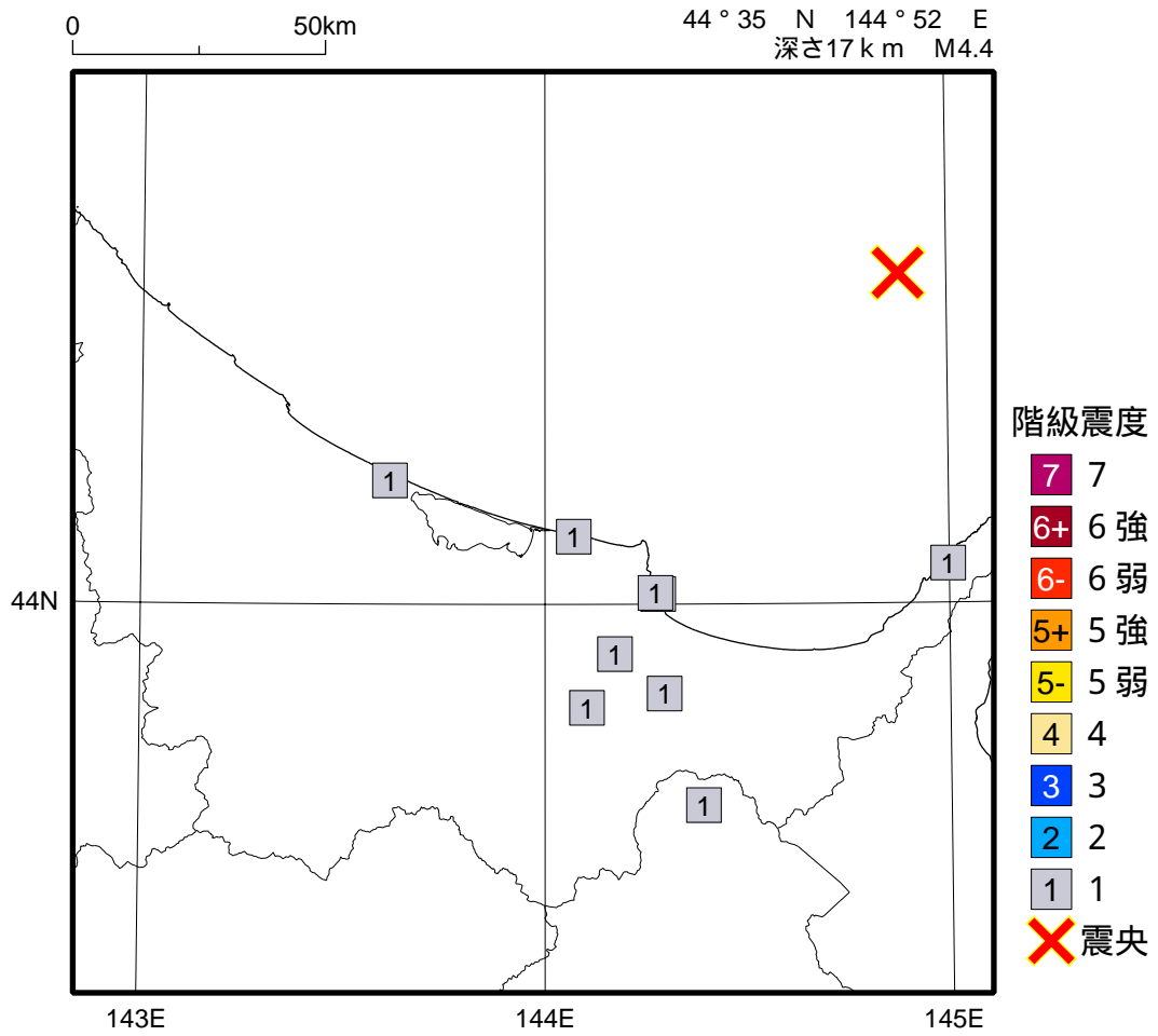
2021年 8月21日14時34分 網走沖の地震の震度分布図
