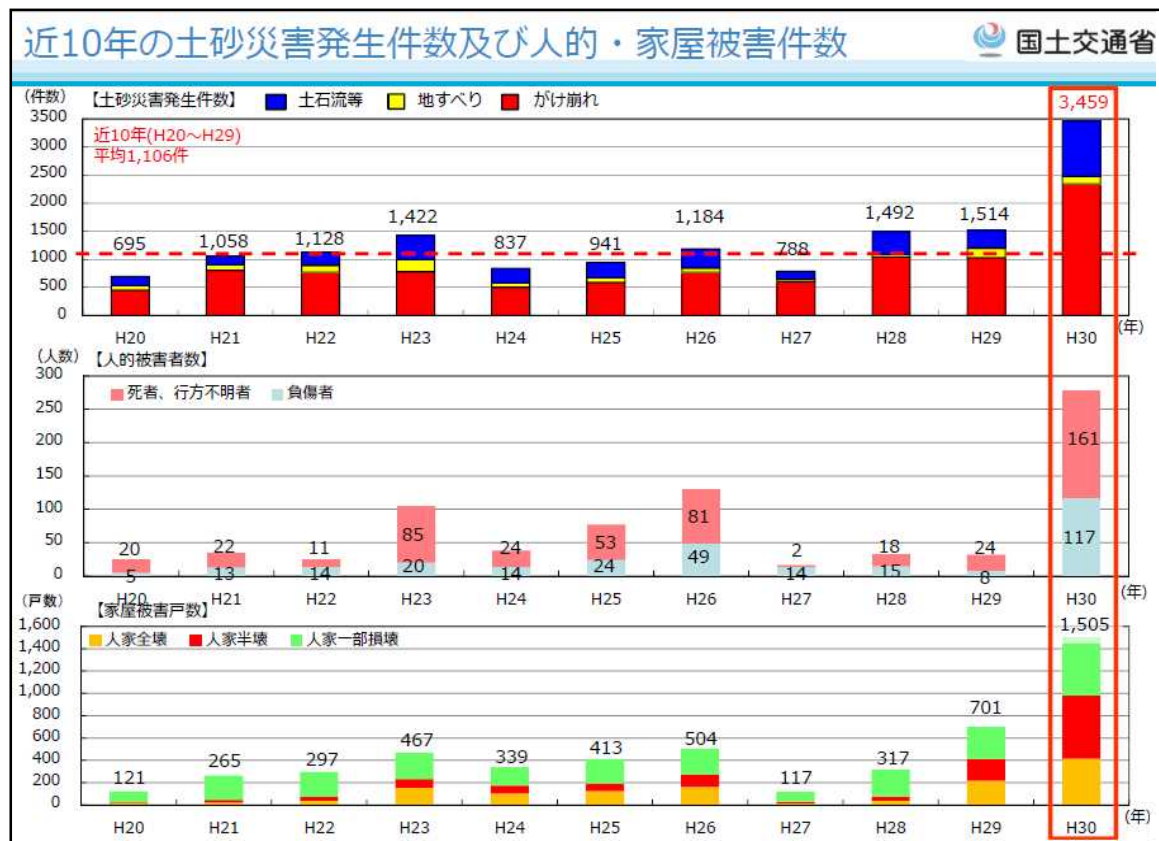
近年の土砂災害発生件数（最近 10 年の年別発生件数）
