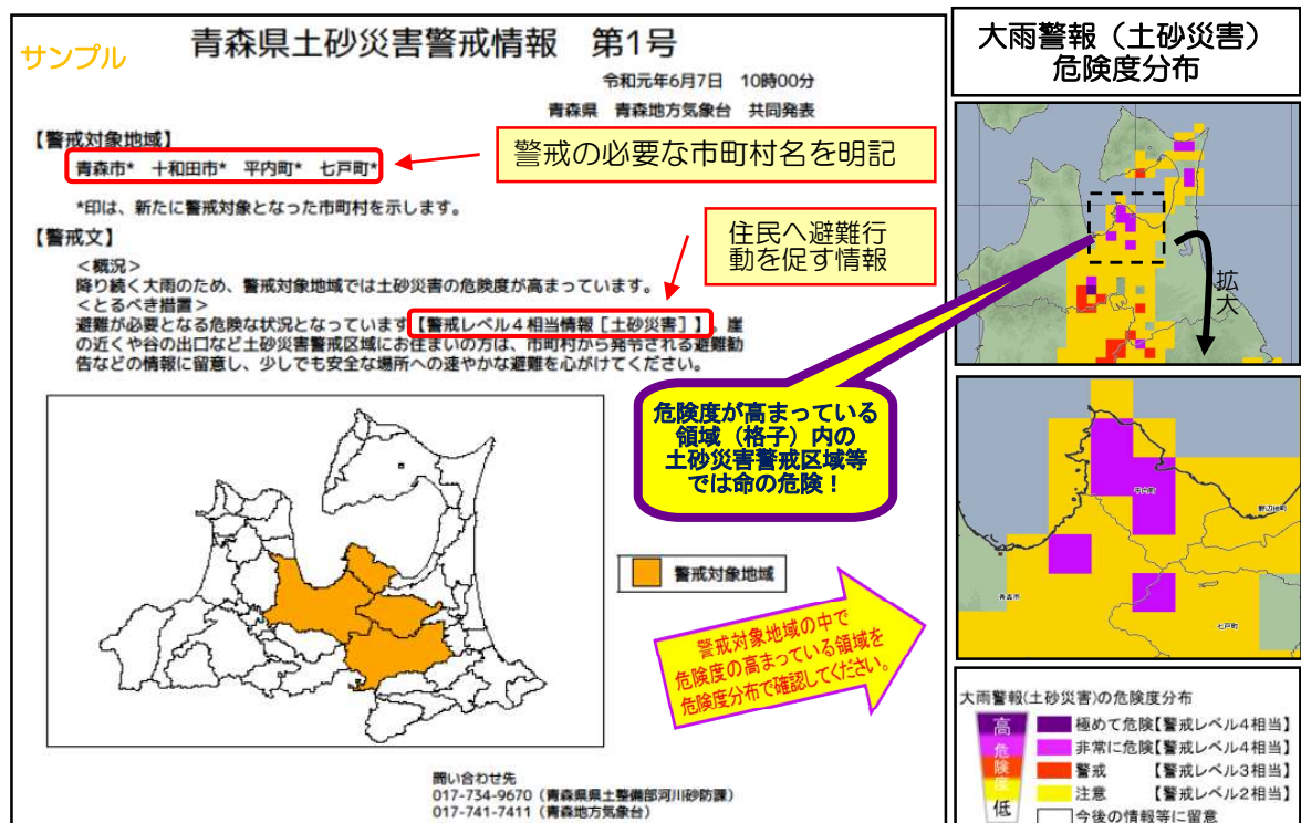
左図：（例）青森県土砂災害警戒情報の発表例
