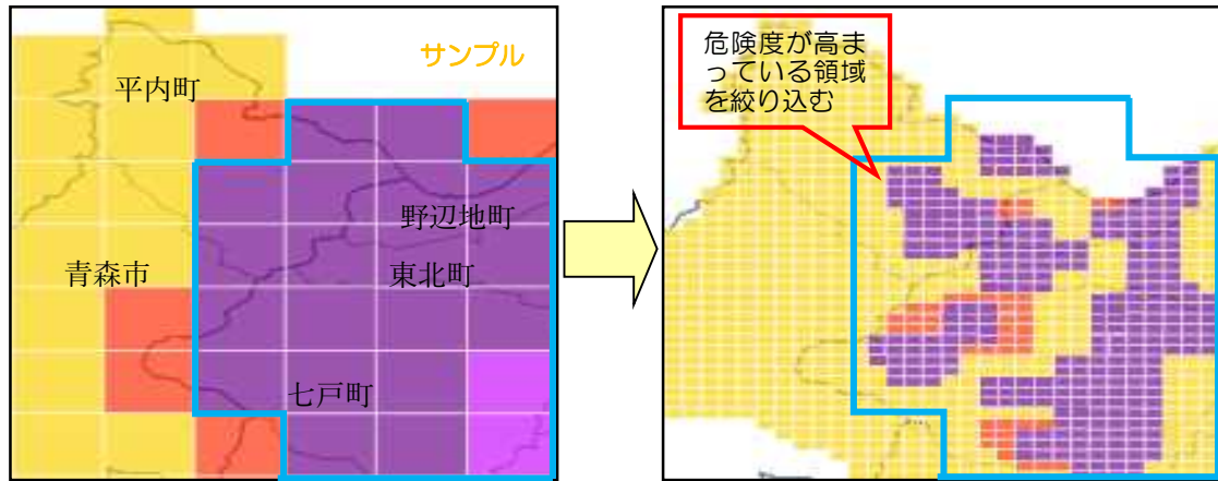
（例）現状の 5km 格子の危険度分布
