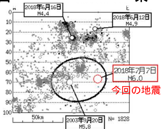
上図の四角形領域内の東西断面図 西 東
