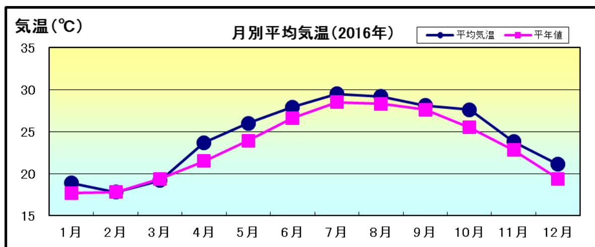
図1 南大東島の月別の平均気温(2016年)と平年値
