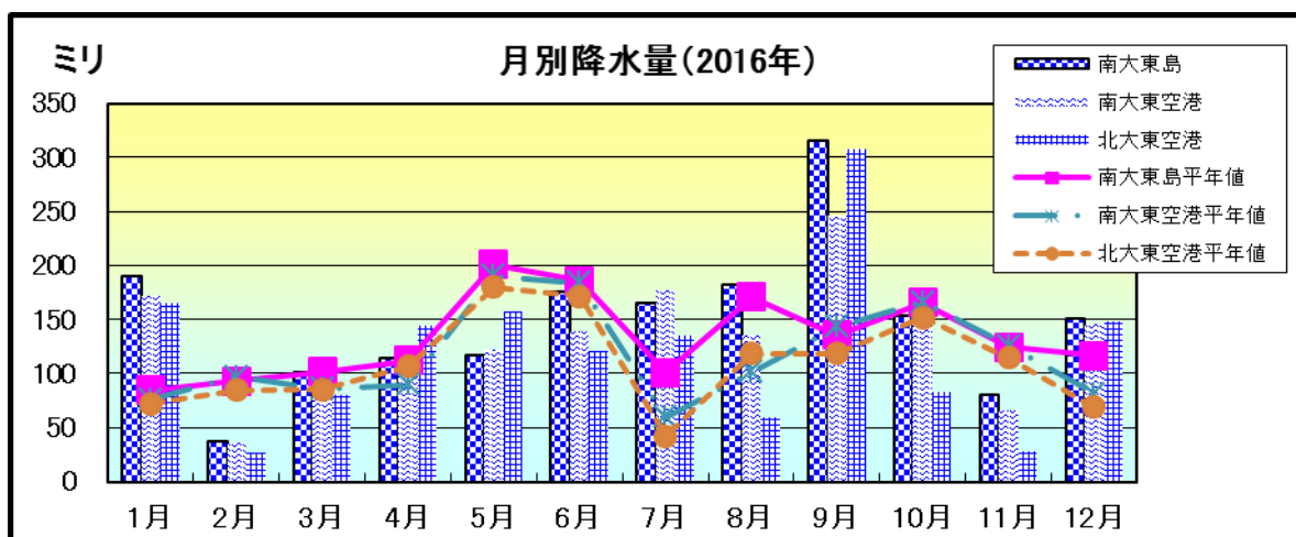
図2 月別の降水量(2016年)と平年値
