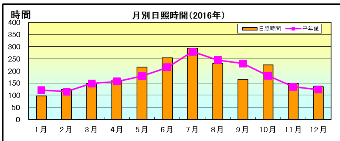
図3 南大東島の月別の日照時間(2016年)と平年値
