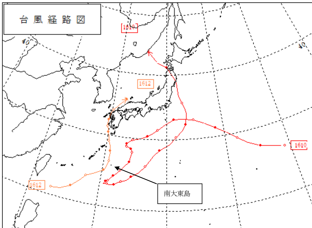
図4 大東島地方に接近した台風の経路図(2016年)
