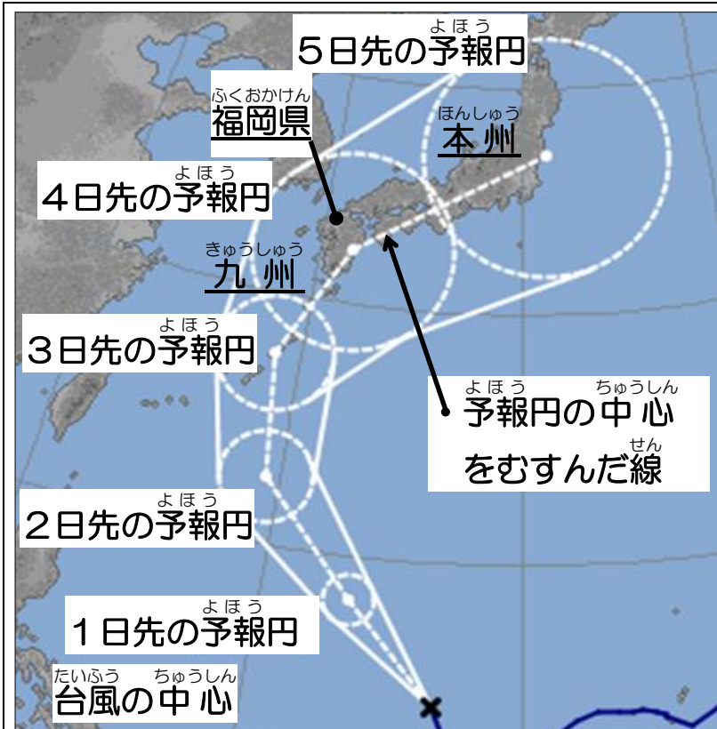
図 5日進路予報
