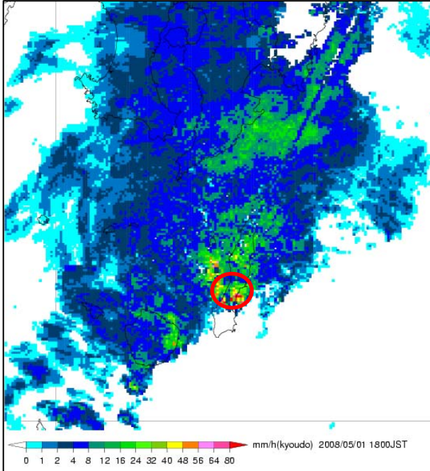
5月1日17時50分のレーダー画像
