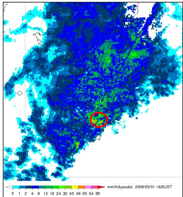
5月1日18時20分のレーダー画像
