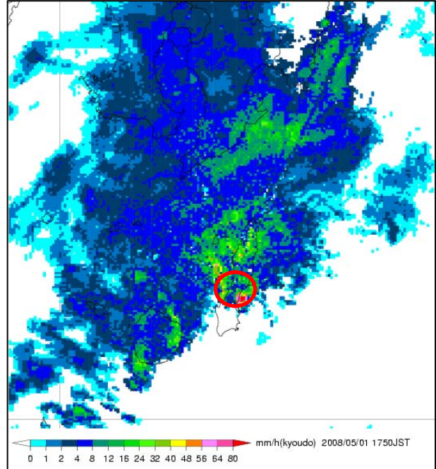
5月1日18時00分のレーダー画像
