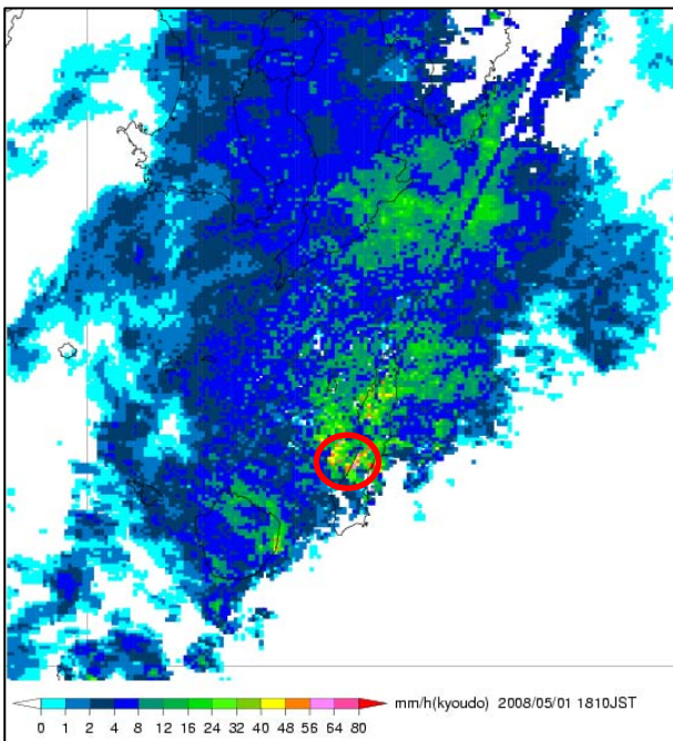
5月1日18時10分のレーダー画像
