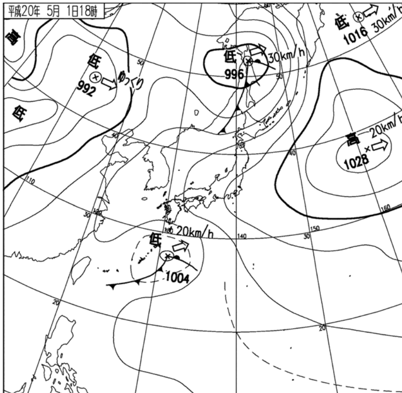
平成 20 年 5 月 1 日 18 時の地上天気図
