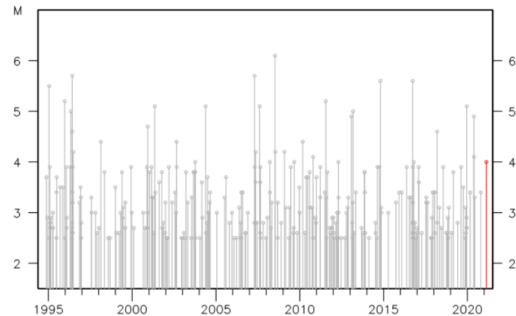
領域b内の地震活動経過図
