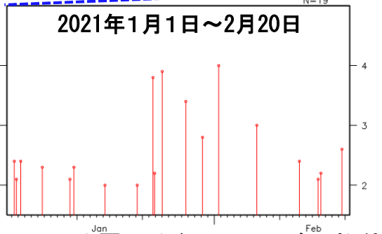
震域a内の地震活動経過図及び回数積算図
