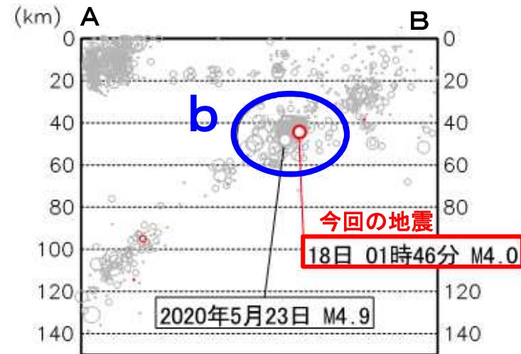
領域a内の断面図
