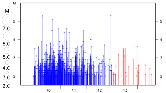
左図領域 a 内の地震活動経過図
