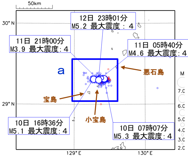
震央分布図
