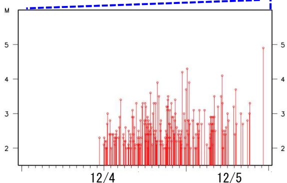
左図領域a内の地震活動経過図 (上図：1994年10月1日~2021年12月5日12時 下図：2021年12月4日00時~2021年12月5日12時、M \geq 2.0)
