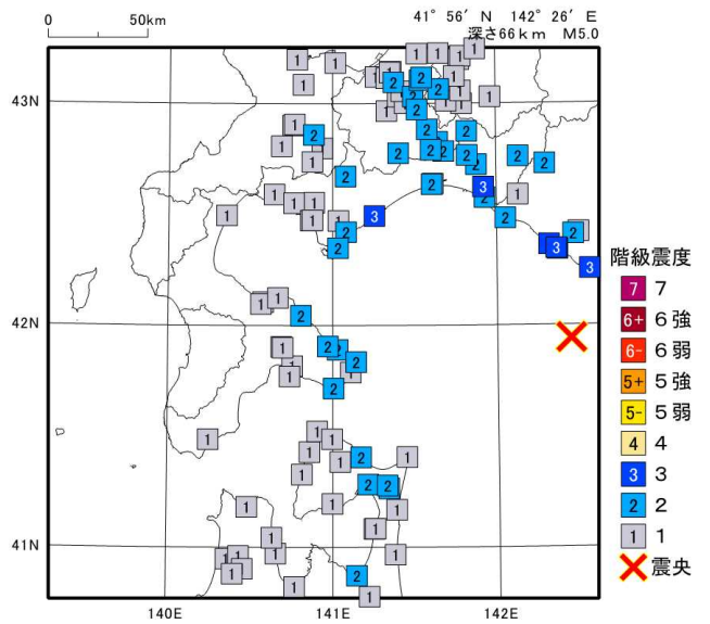
2024年 4月 5日05時31分 浦河沖の地震の震度分布図
