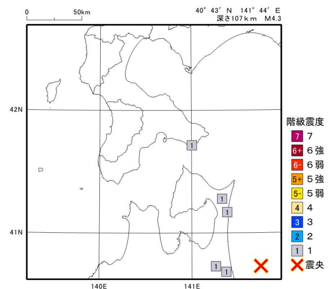
2024年 4月11日16時13分 青森県東方沖の地震の震度分布図
