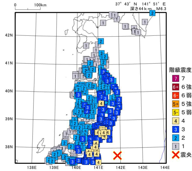
2024年 4月 4日12時16分 福島県沖の地震の震度分布図
