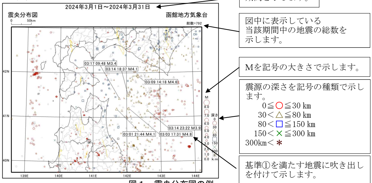
図1 震央分布図の例
