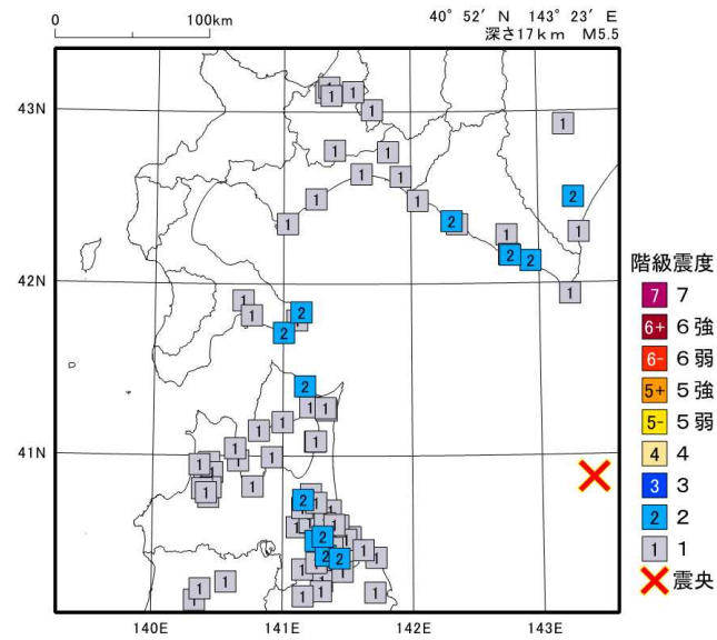
2024年 4月 6日09時12分 青森県東方沖の地震の震度分布図
