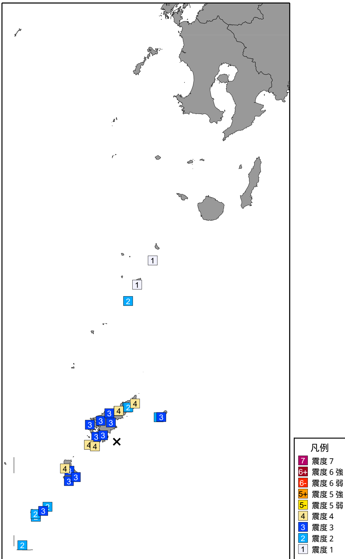
観測点別震度分布図(xは震央)
