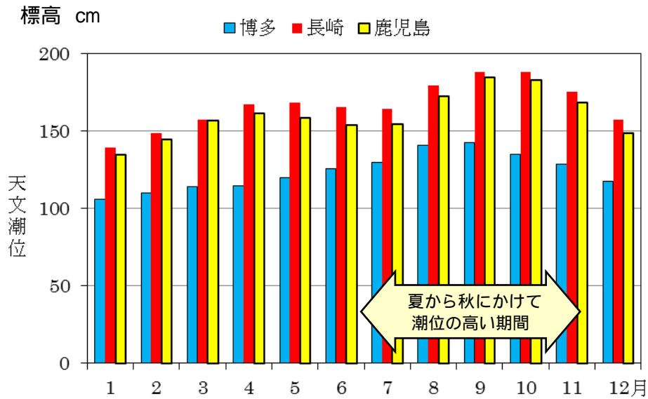
図1 博多・長崎・鹿児島における2016年の各月最高の天文潮位 天文潮位：月と太陽の運行などをもとに計算した潮位の予測値
