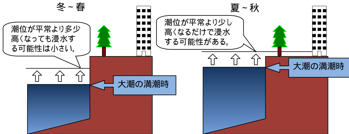
図3 冬～春の潮位と夏～秋の潮位の比較 夏から秋にかけて、大潮の満潮時には潮位が特に高くなる。
