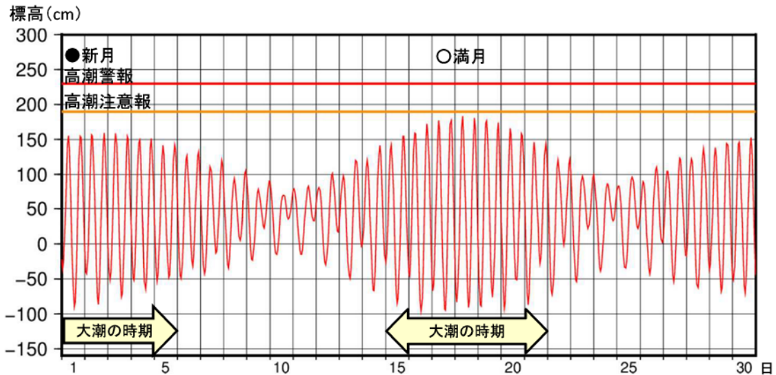
図2 鹿児島における2016年9月の天文潮位 大潮（満月と新月の前後数日）は満潮と干潮の差が大きくなり、満潮時の潮位が特に高くなる。
