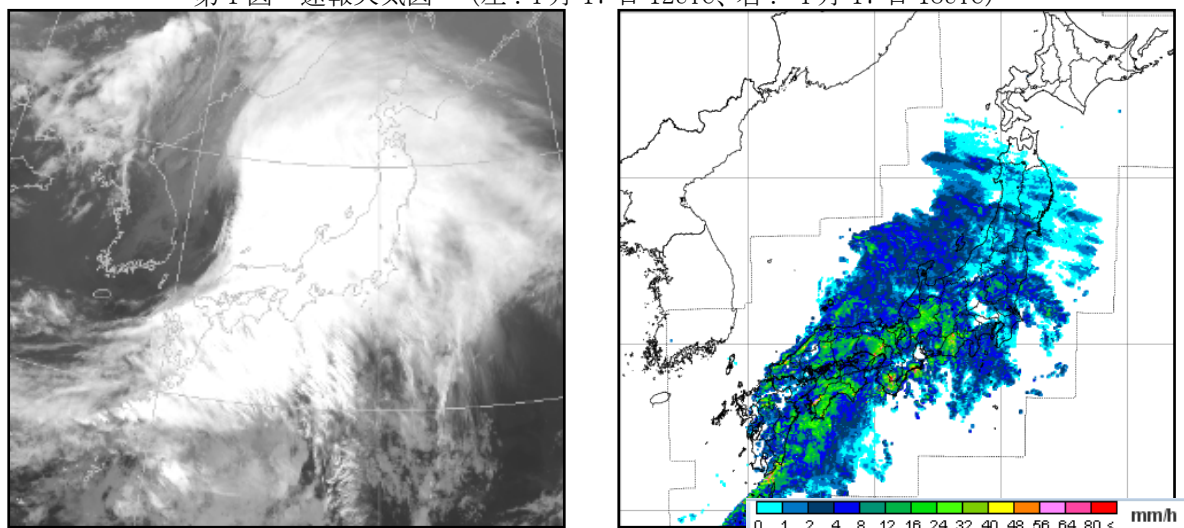
第 2 図 4 月 17 日 12UTC の衛星赤外画像（左）とレーダーエコー分布図（右）
