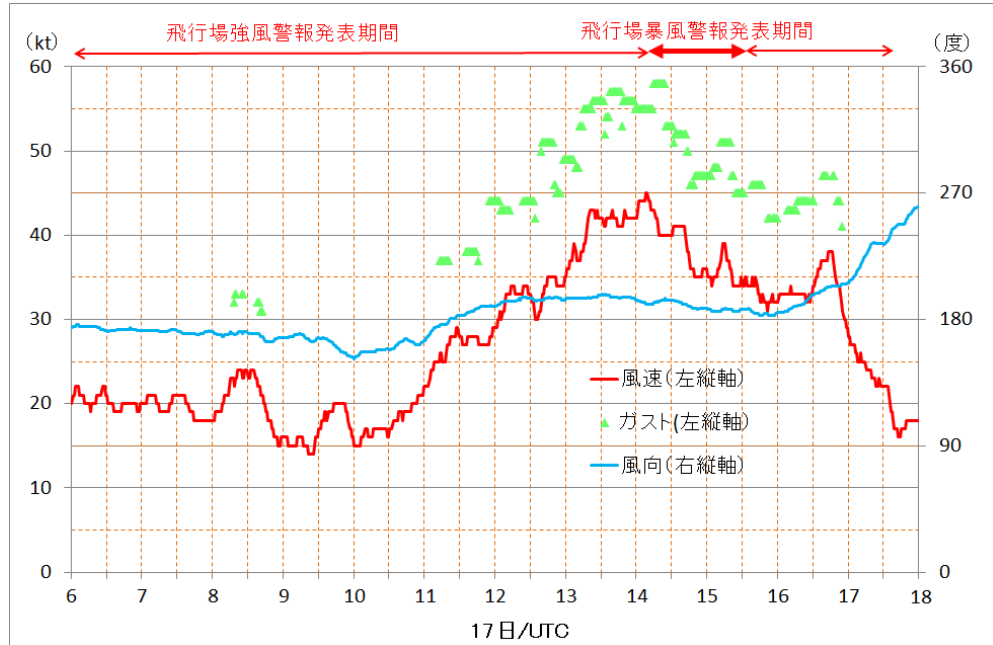
第3図 関西国際空港代表風（06L）の風向と風速（17日06UTC～18UTC）
