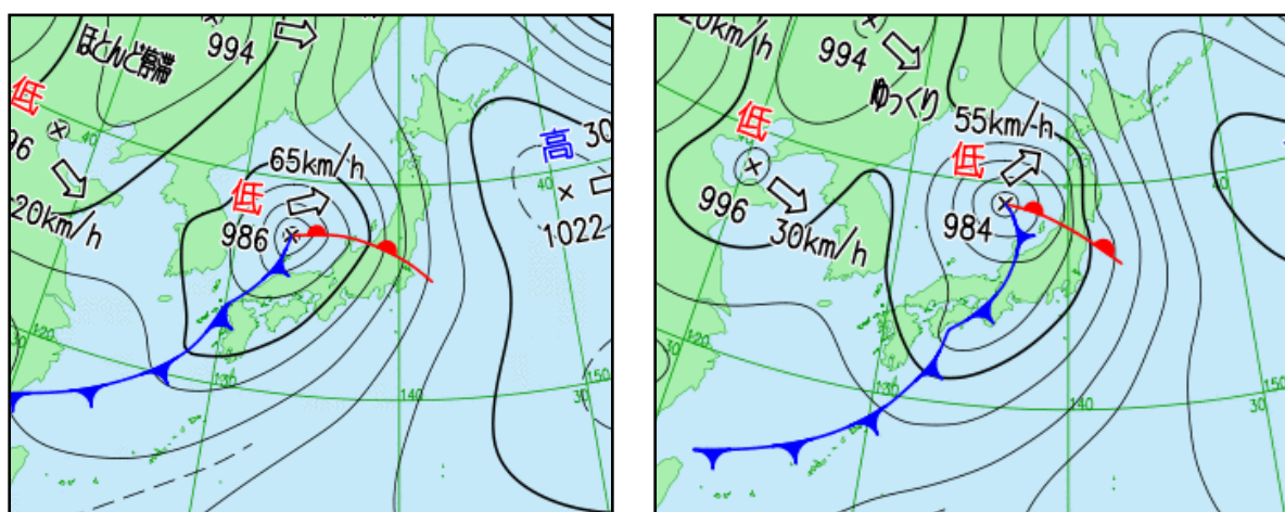
第 1 図 速報天気図（左：4 月 17 日 12UTC、右：4 月 17 日 18UTC）
