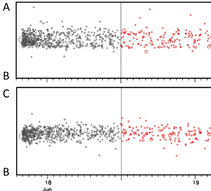
領域a内の時空間分布図(上:A-B投影、下:C-B投影)
