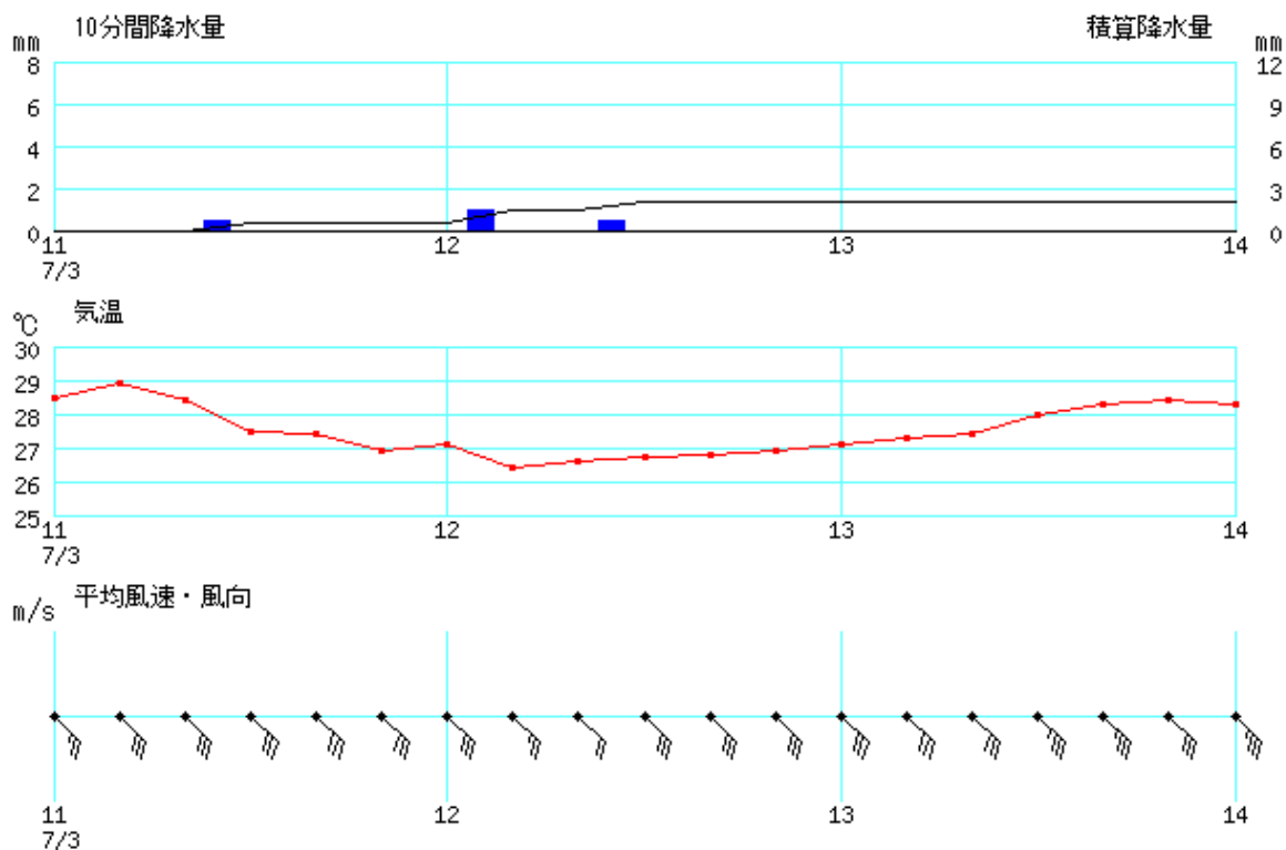
アメダス安芸 時系列グラフ(7月3日11時~14時)
