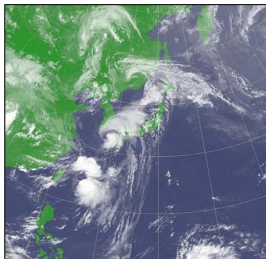
気象衛星赤外画像(7月3日12時)
