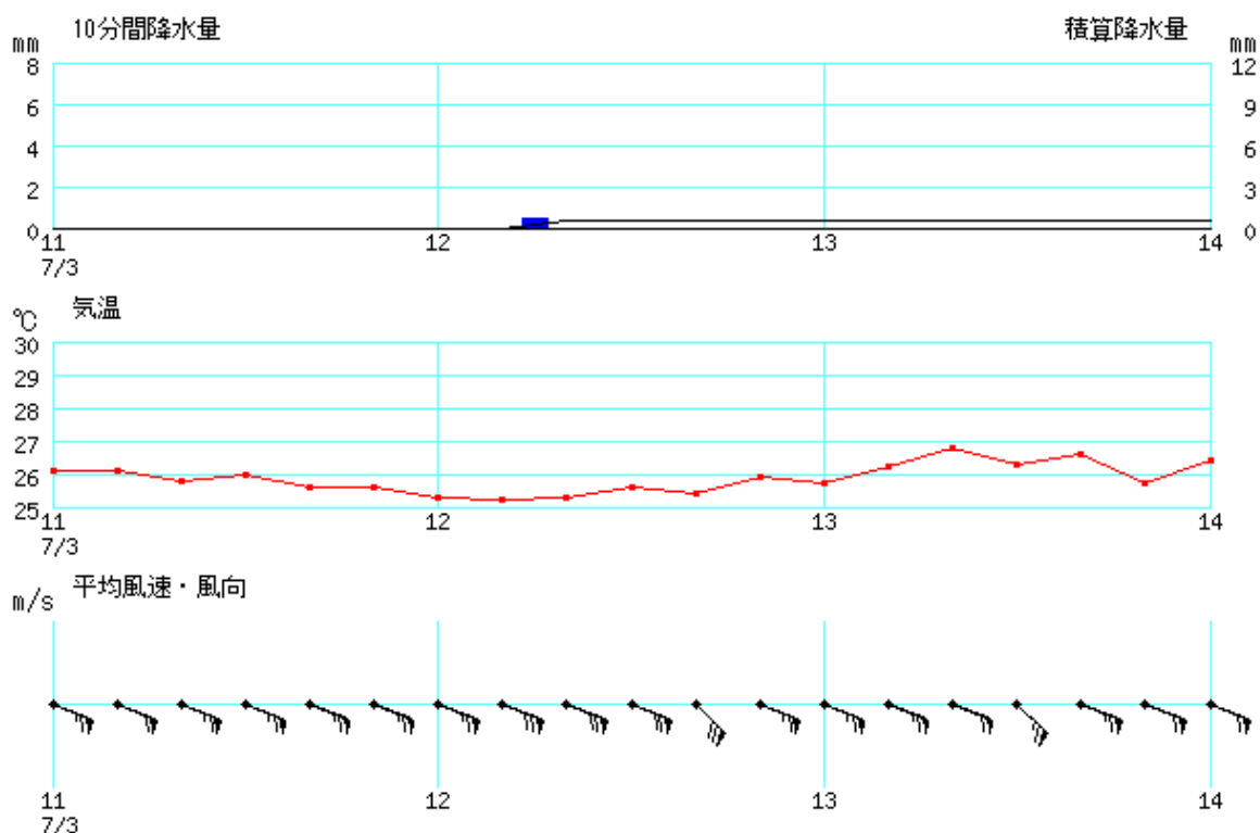
室戸岬特別地域気象観測所 時系列グラフ(7月3日11時~14時)
