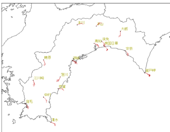
アメダス地点における前10分間平均風向風速分布図 (7月3日12時00分)
