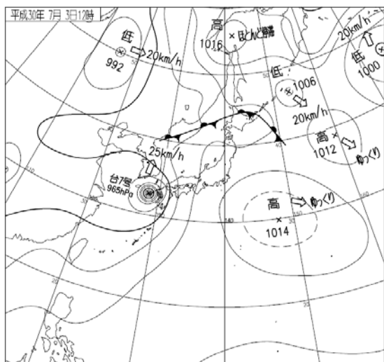
地上天気図(7月3日12時)
