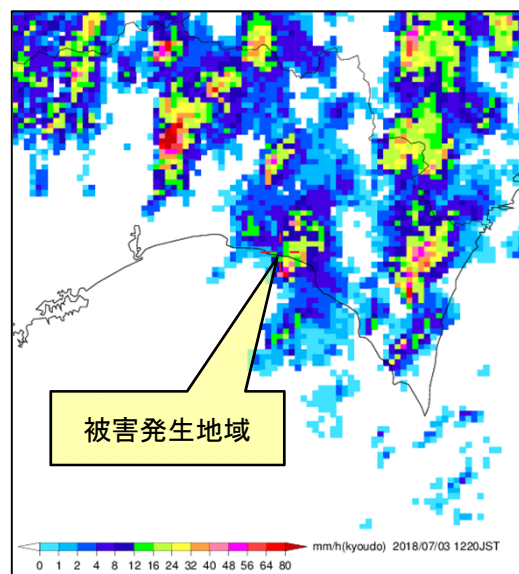
気象レーダー画像(降水強度) (7月3日12時20分)
