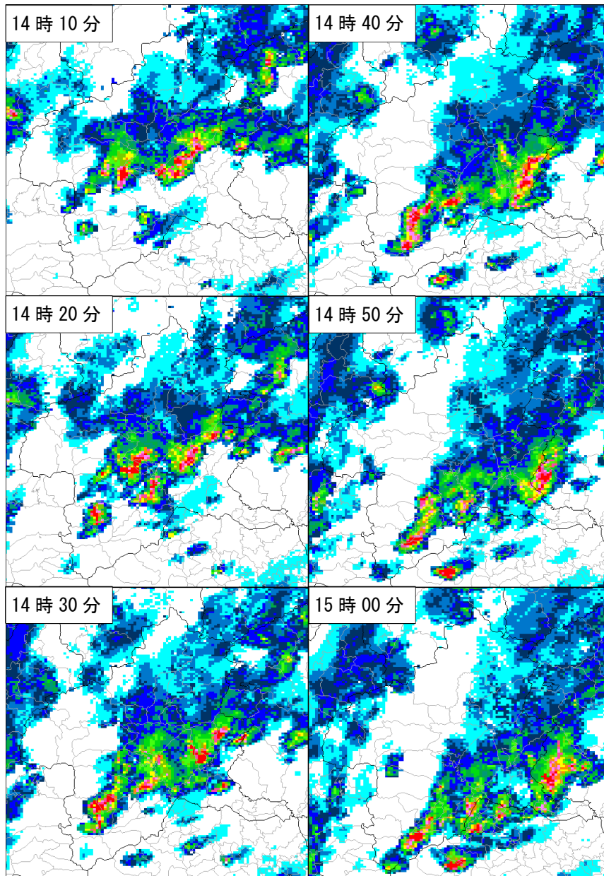
7月11日14時10分から10分毎のレーダー画像
