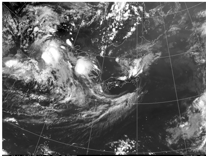
7月11日15時の地上天気図(左)と気象衛星赤外面像(右)
