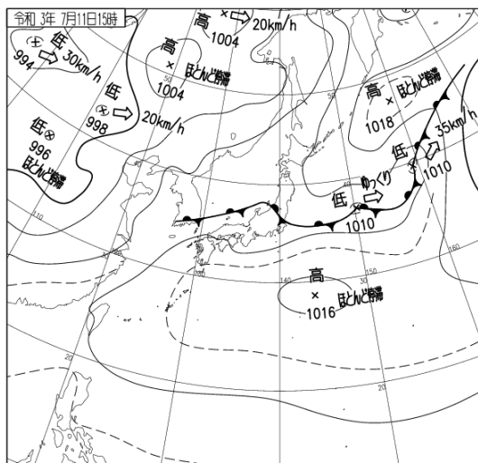
7月11日15時の地上天気図(左)と気象衛星赤外面像(右)
