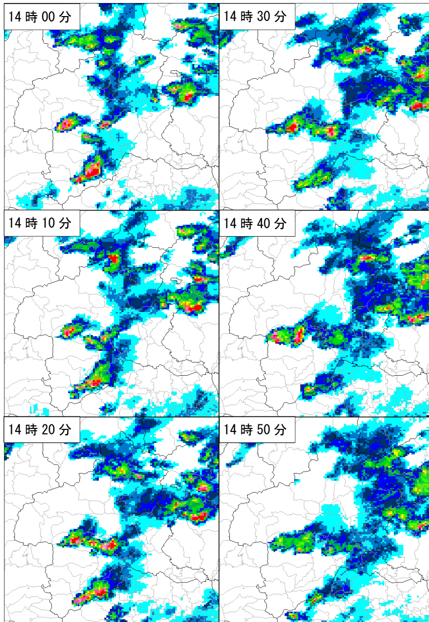
7月12日14時00分から10分毎のレーダー画像
