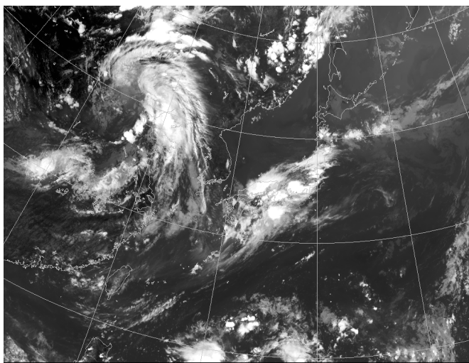
7月12日15時の地上天気図(左)と気象衛星赤外面像(右)
