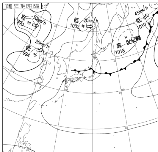
7月12日15時の地上天気図(左)と気象衛星赤外面像(右)
