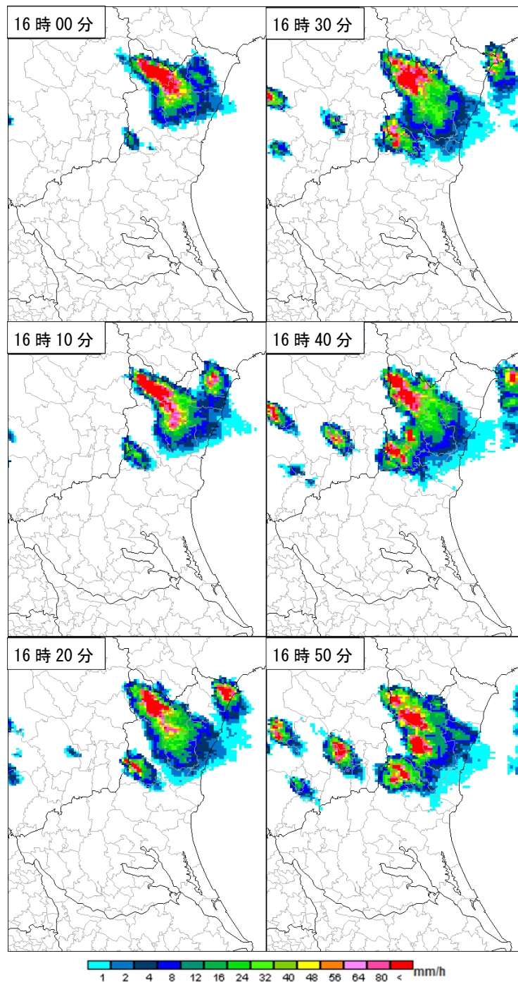
7月16日16時00分から10分毎のレーダー画像
