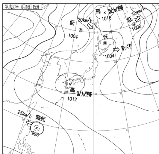
7 月 16 日 15 時の地上天気図（左）と気象衛星赤外面像（右）
