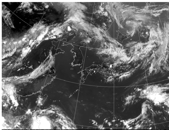
7 月 16 日 15 時の地上天気図（左）と気象衛星赤外面像（右）
