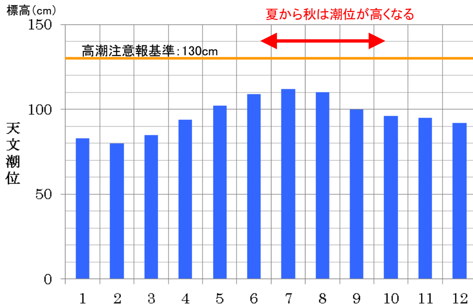
図1. 平良における各月の最高の天文潮位 (平成29年)
