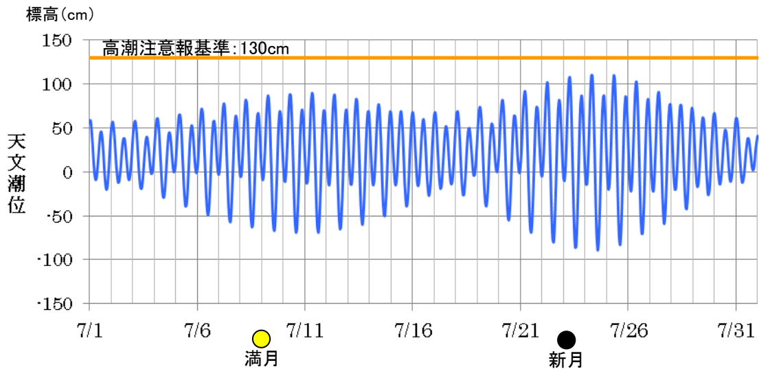
図2. 平良における平成29年7月の天文潮位の変化 満月または新月の前後数日間 (大潮の時期) は満潮時の潮位が特に高くなる。
