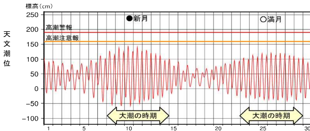
図3 博多における2018年9月の天文潮位
