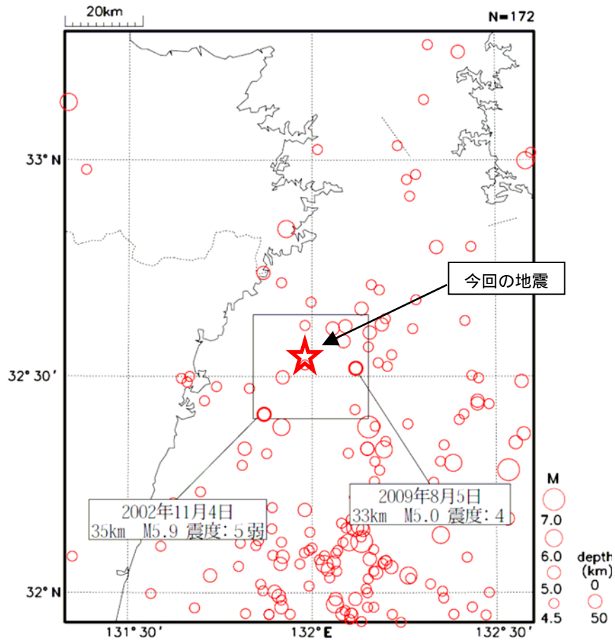
日向灘を震源とする地震の震央分布図 (1923年8月以降、深さ0~50km、M 4.5)
