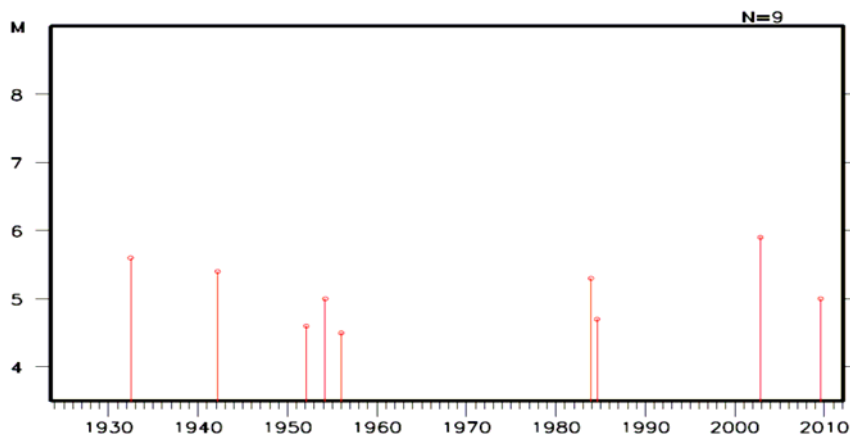
上図矩形内の地震活動経過図
