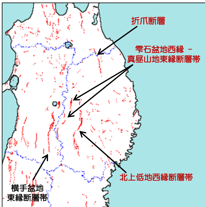
岩手県の活断層
