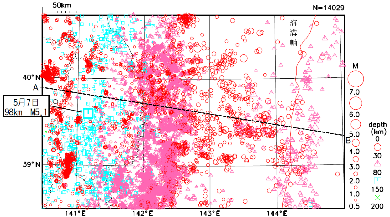
図 1. 2018 年の岩手県とその周辺の震央分布図
