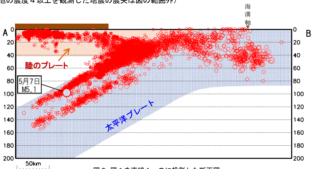
図 2. 図 1 を直線 A-B に投影した断面図
