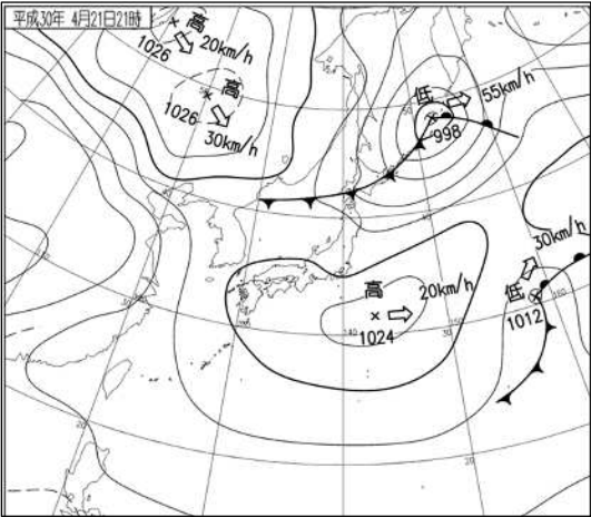
実況天気図 4月21日 21時
