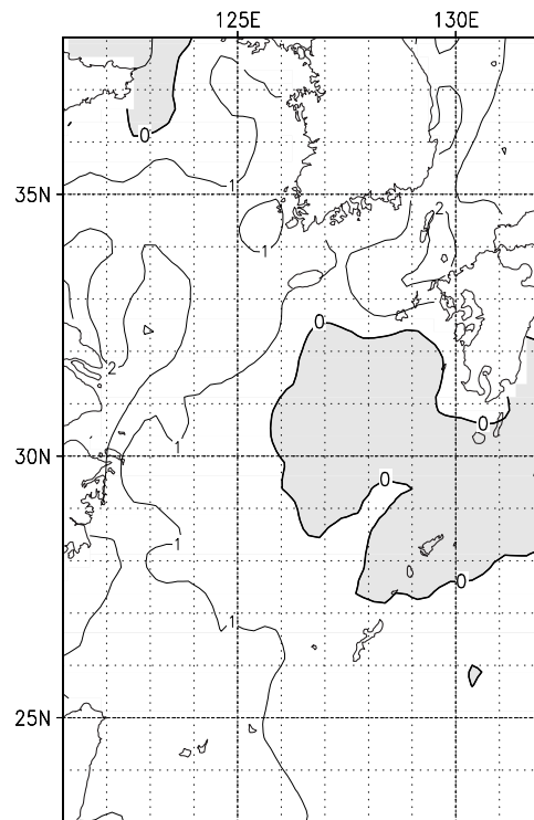
2010 年 8 月中旬の旬平均海面水温前年差 (単位:°C)
