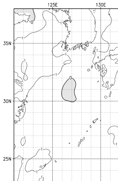
2010 年 8 月中旬の旬平均海面水温平年差 (単位:°C)
