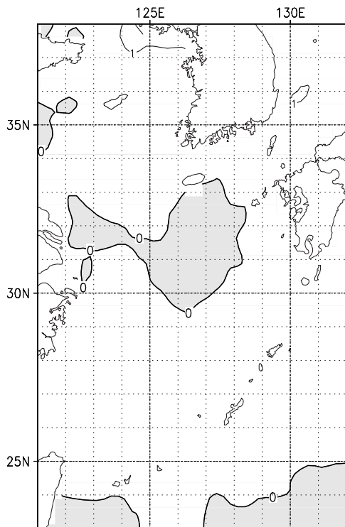
2010 年 8 月中旬の旬平均海面水温前旬差 (単位:°C)
