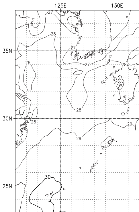
2010 年 8 月中旬の旬平均海面水温 (単位:°C)
