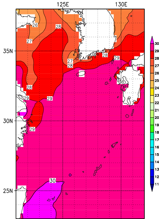
2010年8月下旬の旬平均海面水温 (単位:°C)
