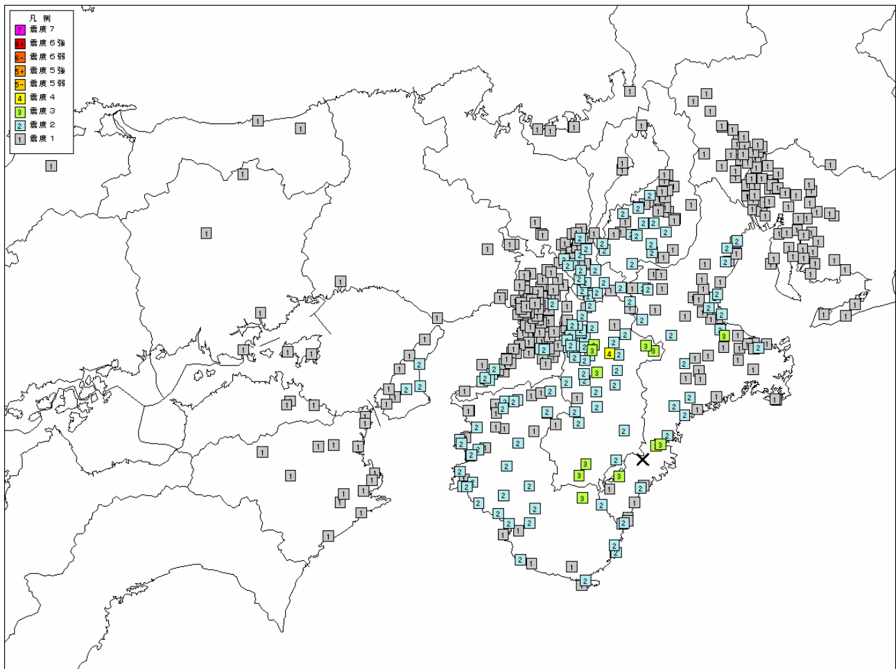
震度分布図（観測点震度） ×印は震央
