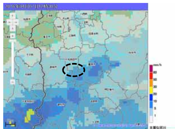
レーダー画像 (4月7日12時30分) ○：被害地域
