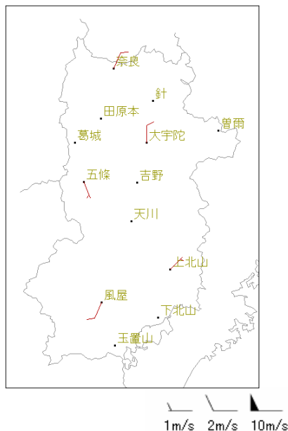
アメダス地点における風向風速分布図 (4月7日12時30分)
