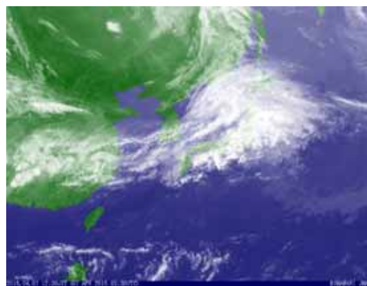
4月7日12時30分の気象衛星赤外画像
