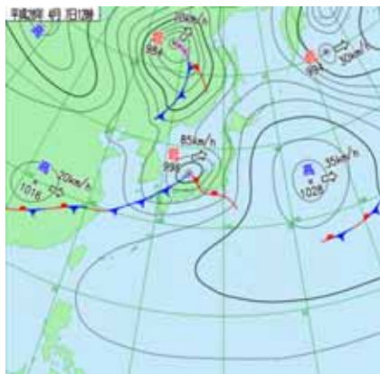
4月7日12時の地上天気図
