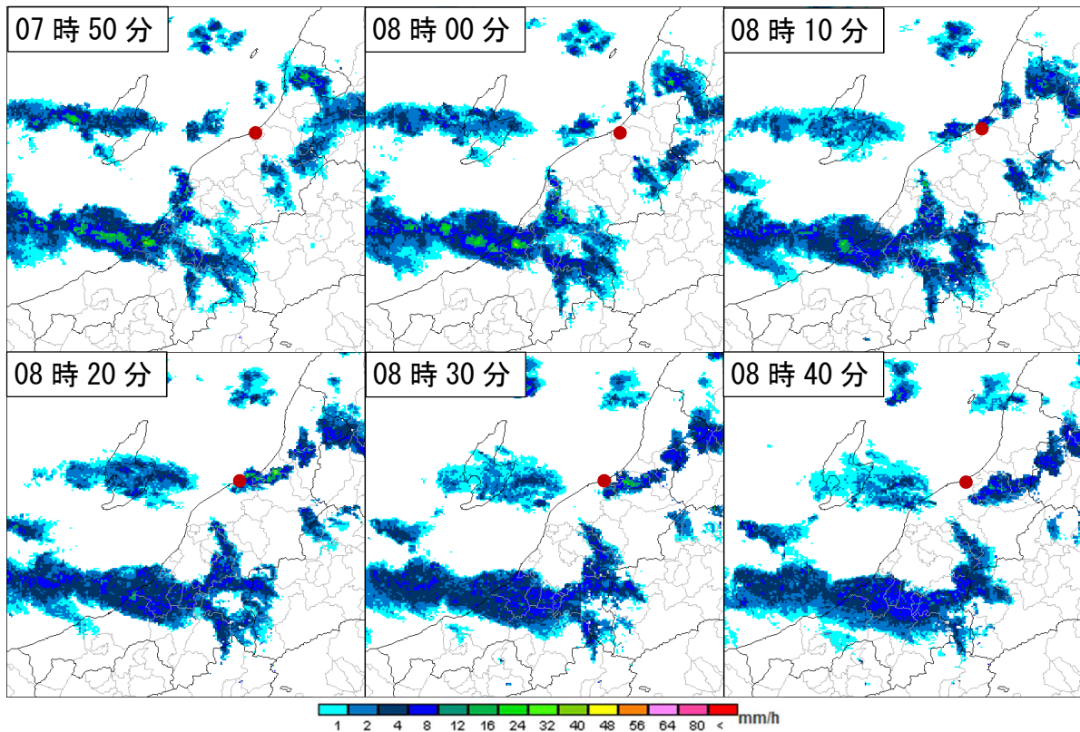
4月2日07時50分から10分毎のレーダー画像
