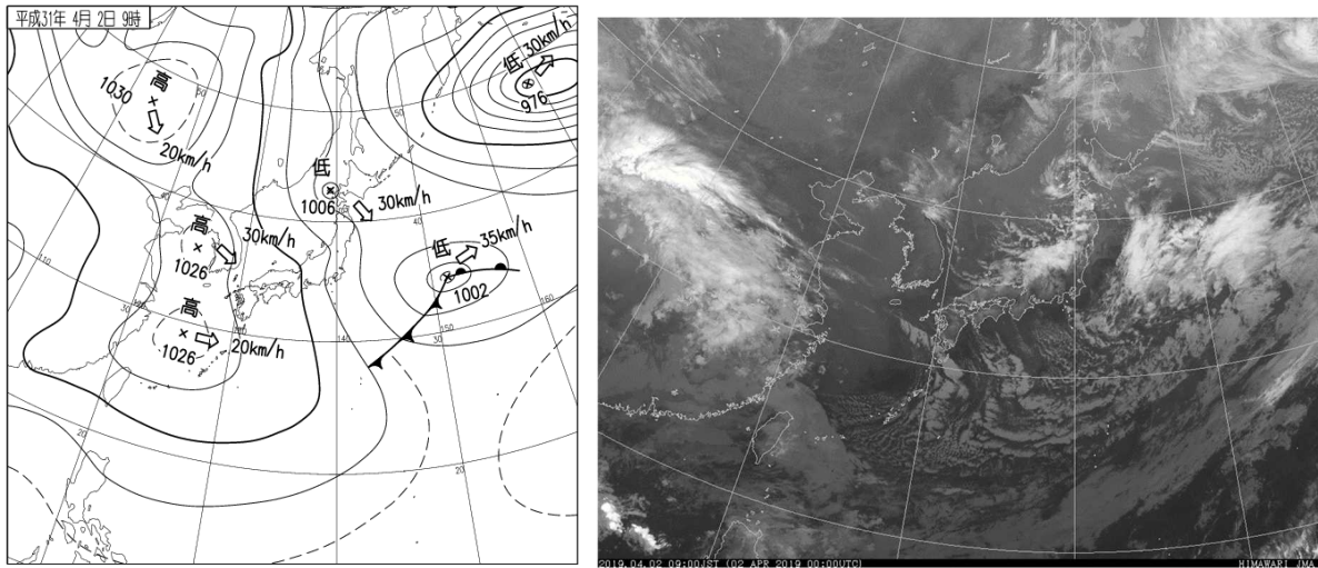
4月2日09時の地上天気図（左）と気象衛星赤外画像（右）
