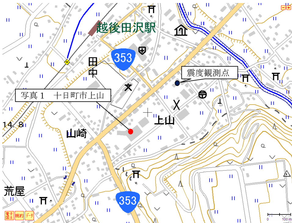
図2 被害状況調査地域周辺図 (新潟県十日町市上山)
