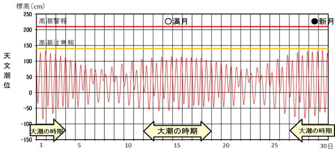
図3 大分における2019年9月の天文潮位
