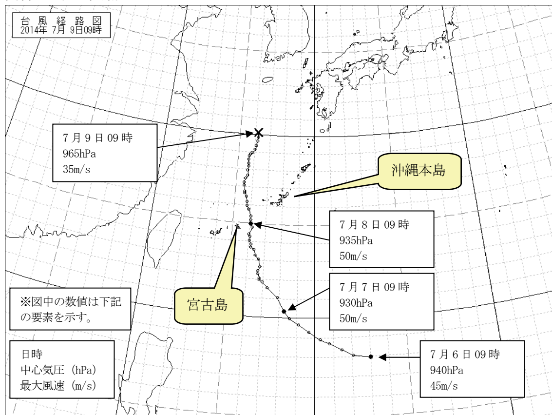
台風第8号経路図（2014年7月9日09時現在 速報値）
