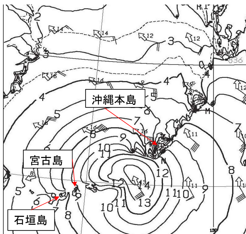
沿岸波浪実況図 2014年7月8日09時
