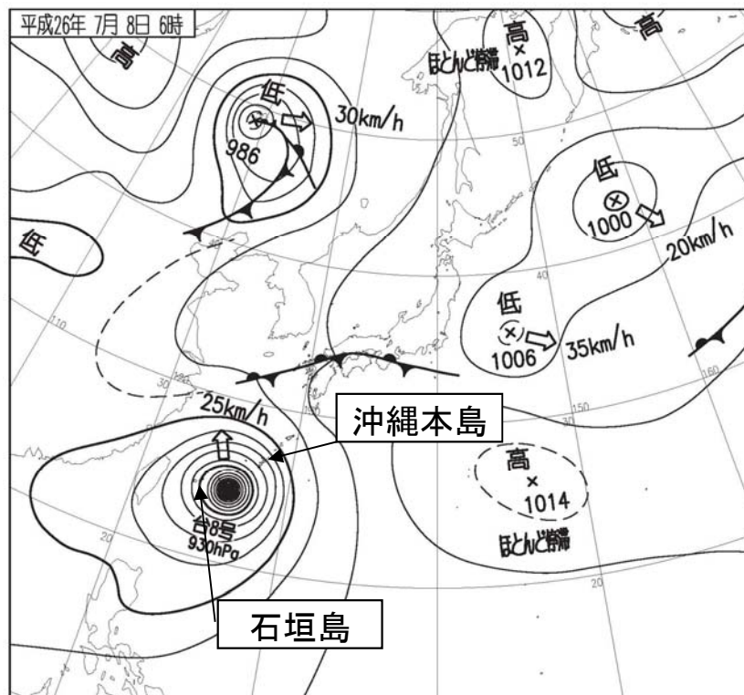
地上天気図 2014年7月8日06時
