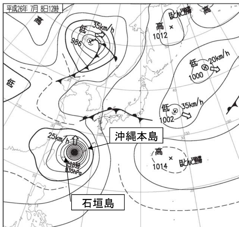
地上天気図 2014年7月8日12時
