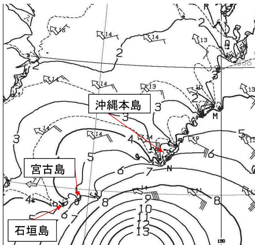
沿岸波浪実況図 2014年7月7日21時
