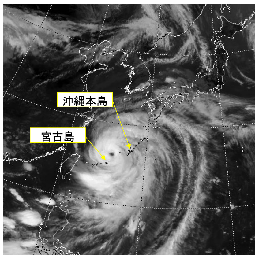
気象衛星画像（赤外）2014年7月8日12時
