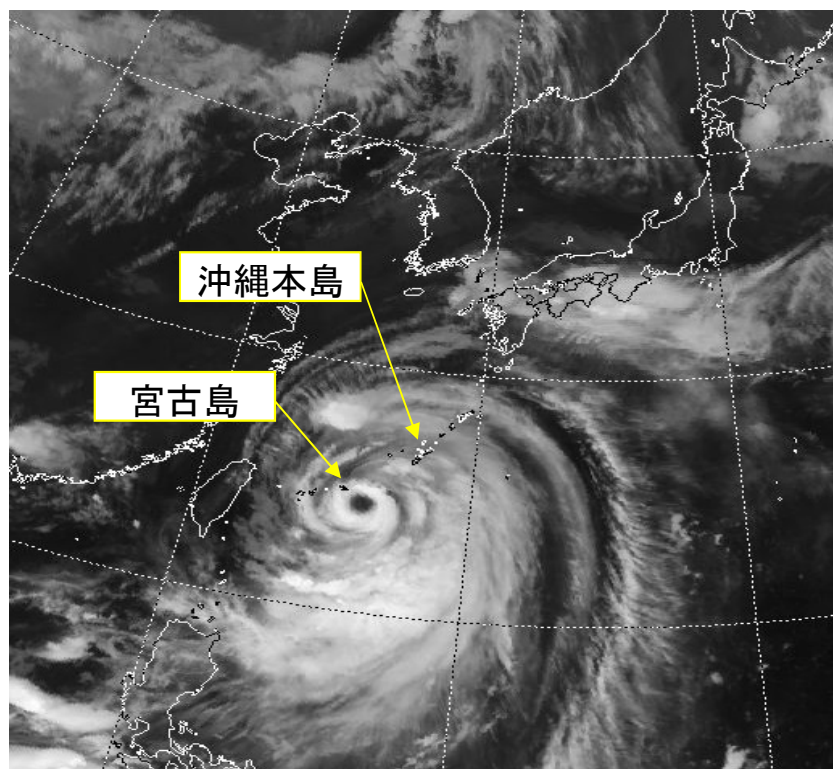
気象衛星画像（赤外）2014年7月8日06時
