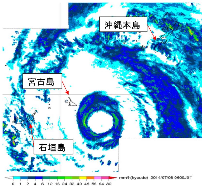
気象レーダー（降水強度）2014年7月8日06時
