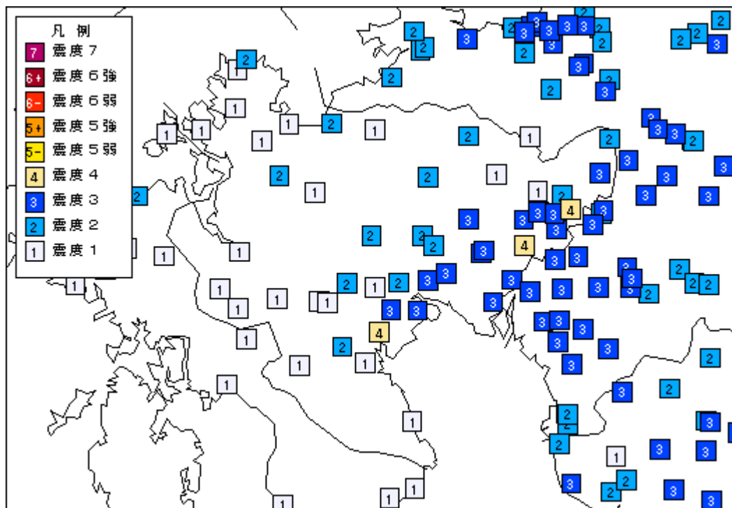
3月14日02時07分頃の地震の震度分布図（佐賀県付近の拡大図）
