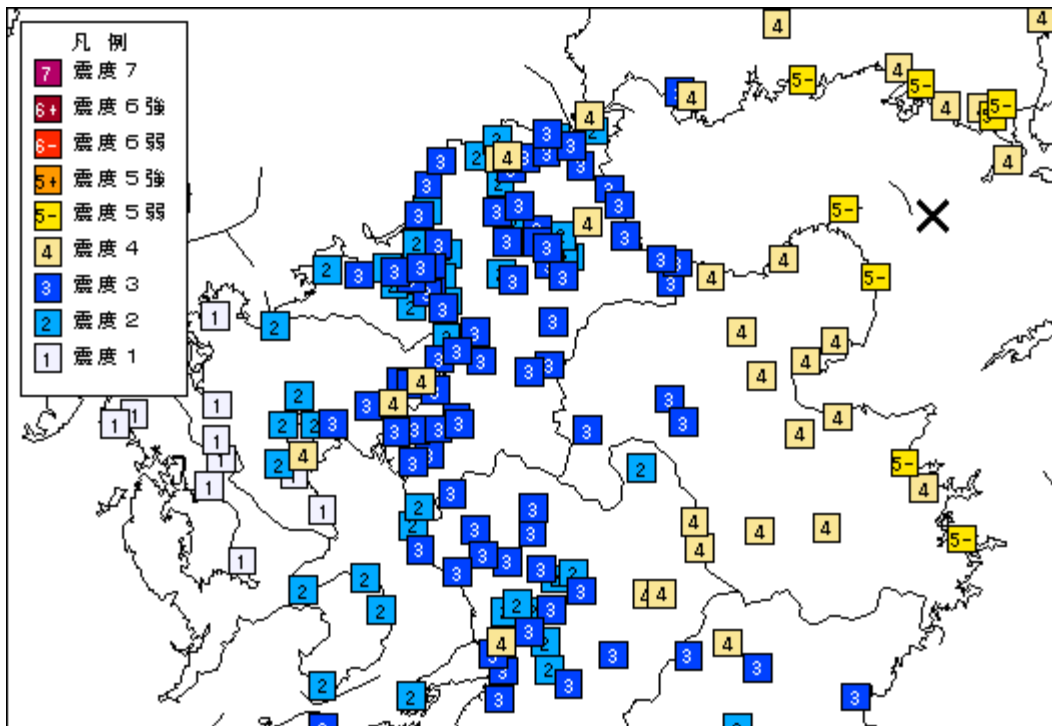
3月14日02時07分頃の地震の震度分布図
