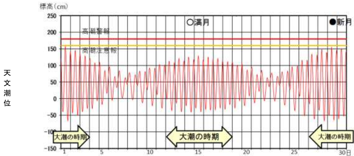
図3 唐津における2019年9月の天文潮位
