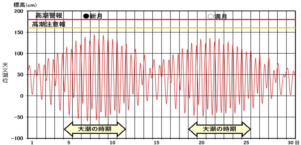
図3 唐津における2021年9月（1時間ごとの）の天文潮位
