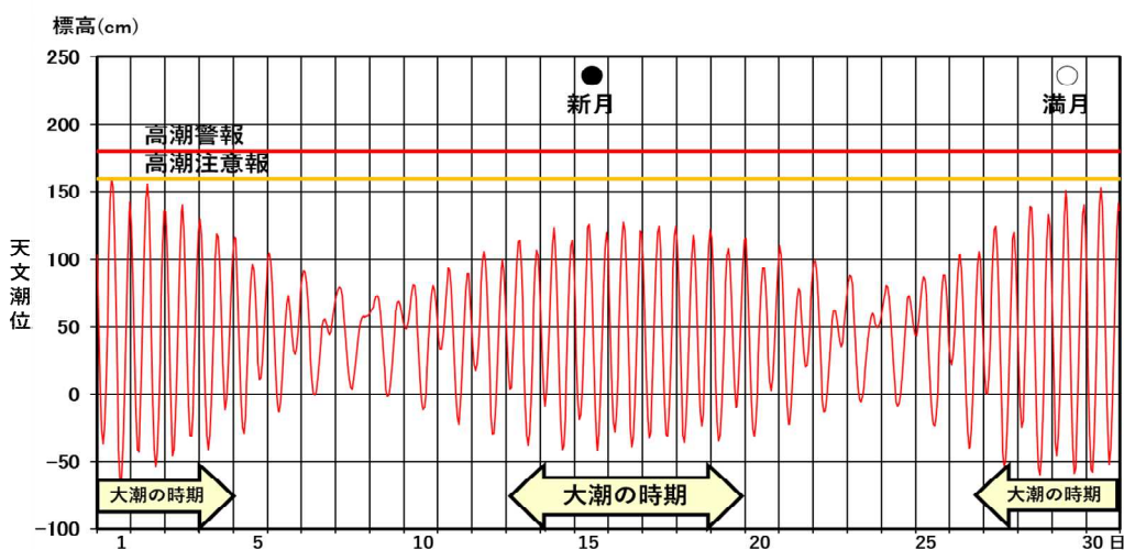
図3 唐津における2023年9月（1時間ごと）の天文潮位
