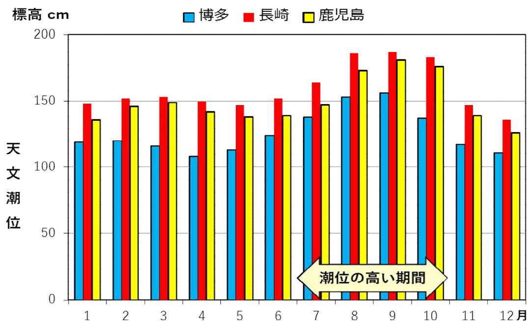
図2 博多・長崎・鹿児島における2023年の各月最高の天文潮位
