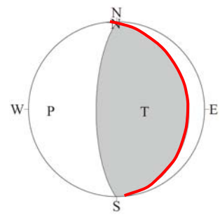
解析に用いたメカニズム解 (USGS CMT 解)
