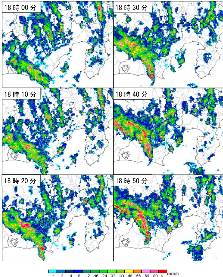
8月23日18時00分から10分毎のレーダー画像
