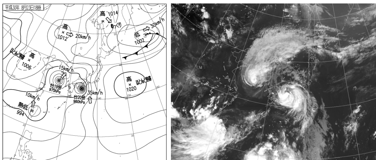
8月23日18時の地上天気図（左）と気象衛星赤外画像（右）
