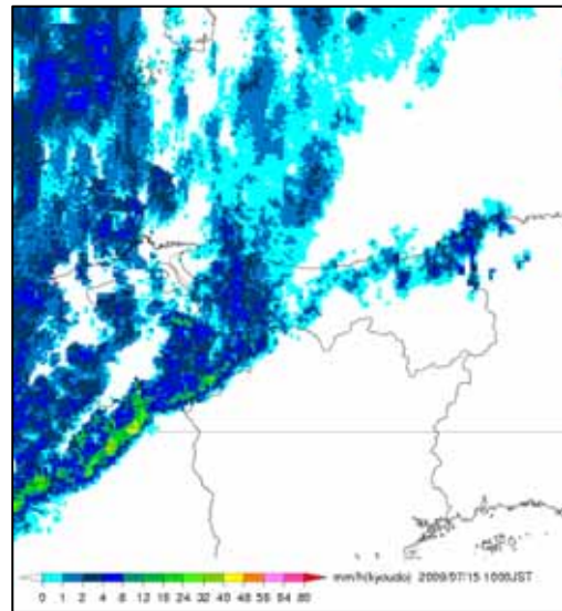
レーダー画像（7月15日09時00分） レーダー画像（7月15日10時00分）
