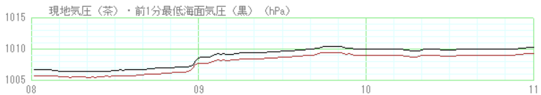
米子特別地域気象観測所：現地気圧時系列グラフ（7月15日08時～11時）
