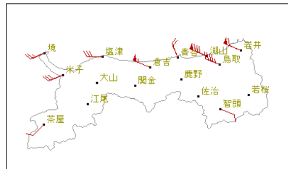
アメダス地点における風向風速分布図 （7月15日10時00分）
