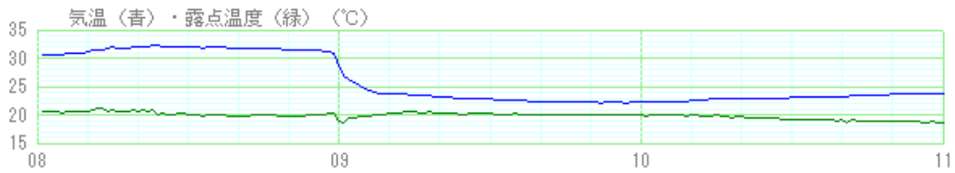
米子特別地域気象観測所：気温・露点温度時系列グラフ（7月15日08時～11時）
