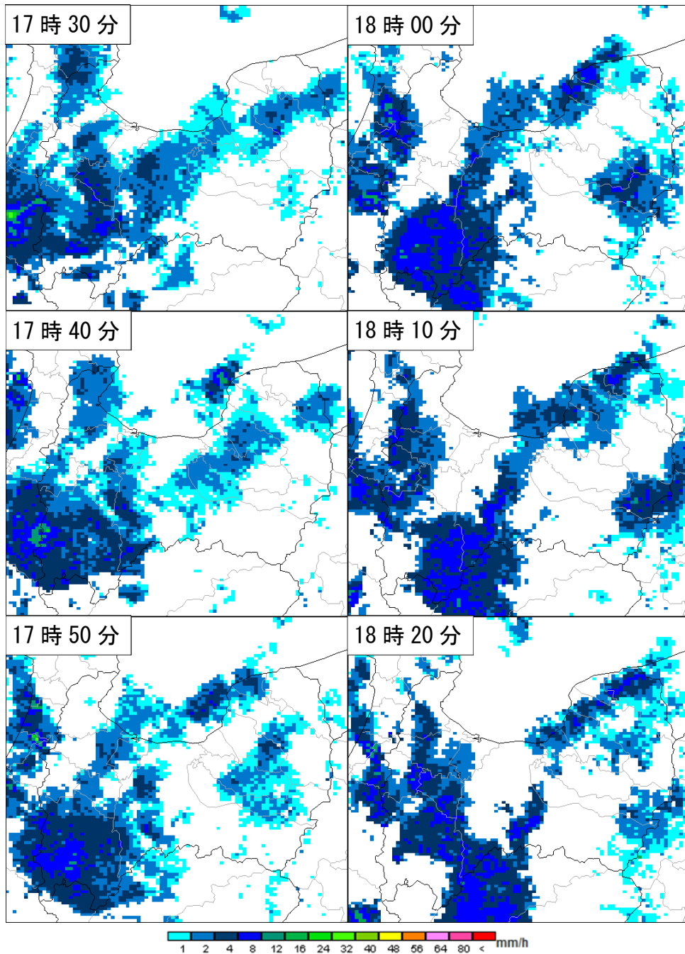
2月4日17時30分から10分毎のレーダー画像
