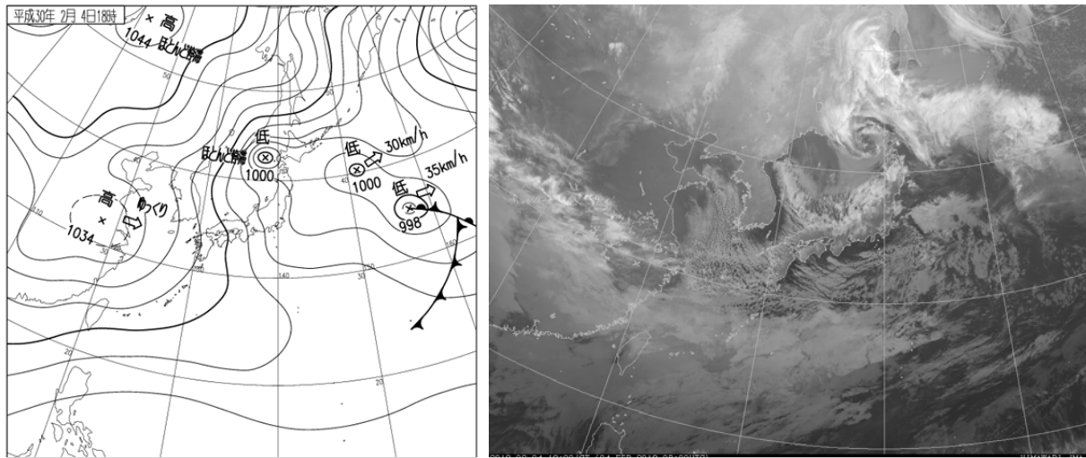
2月4日18時の地上天気図（左）と気象衛星赤外画像（右）
