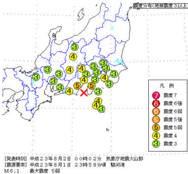
図2 震源位置
