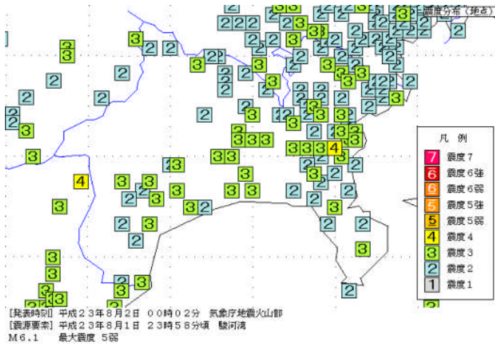
図1 震度分布図
