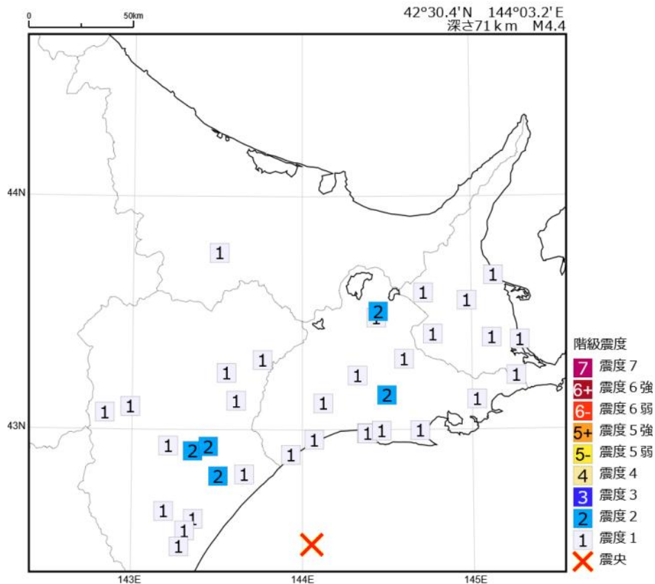
図 4 震度分布図の例
