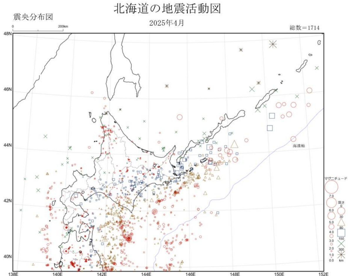
図３ 北海道の震央分布図の例
