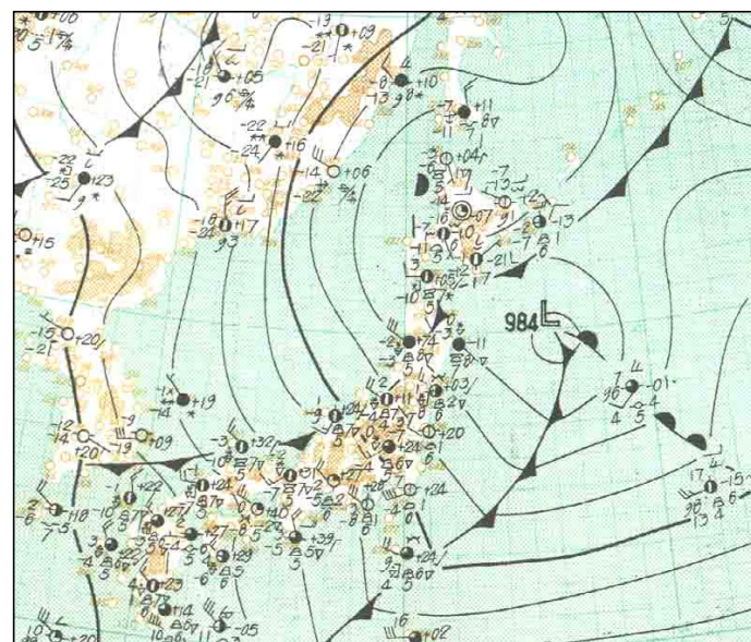
1963年1月19日09時の地上天気図
