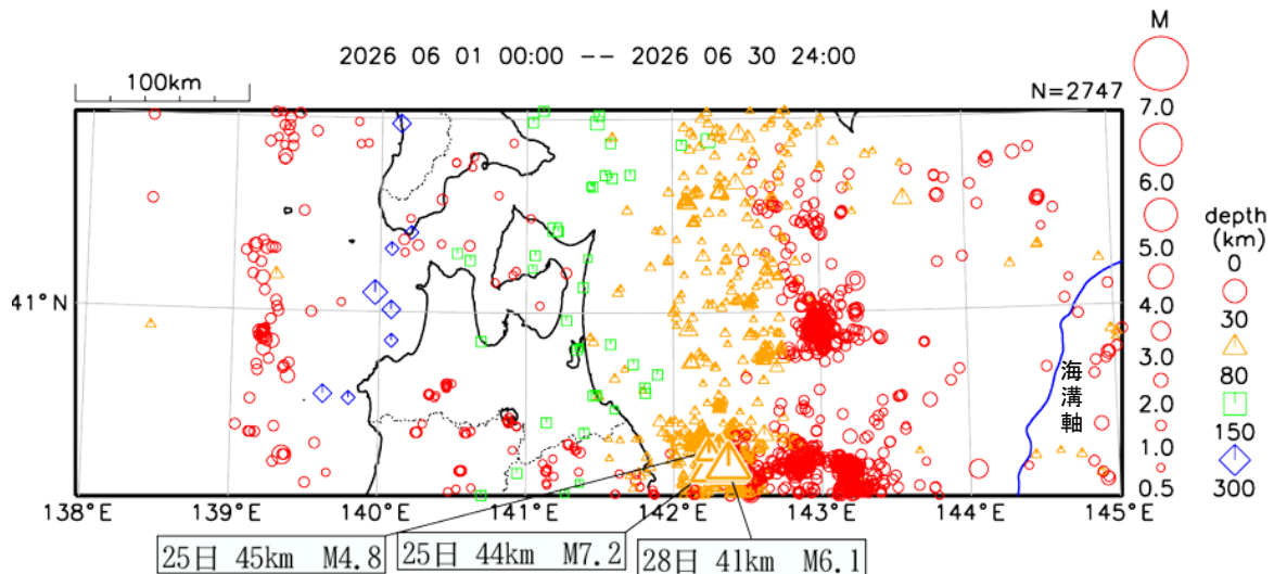
震央分布図
