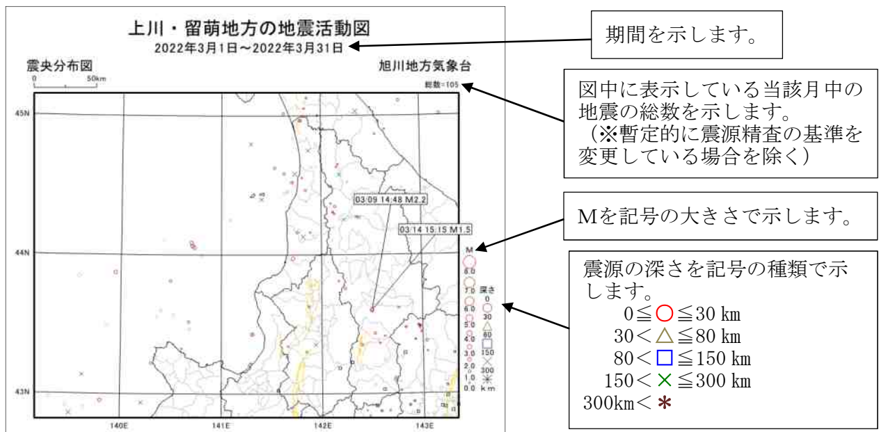
図1 震央分布図
