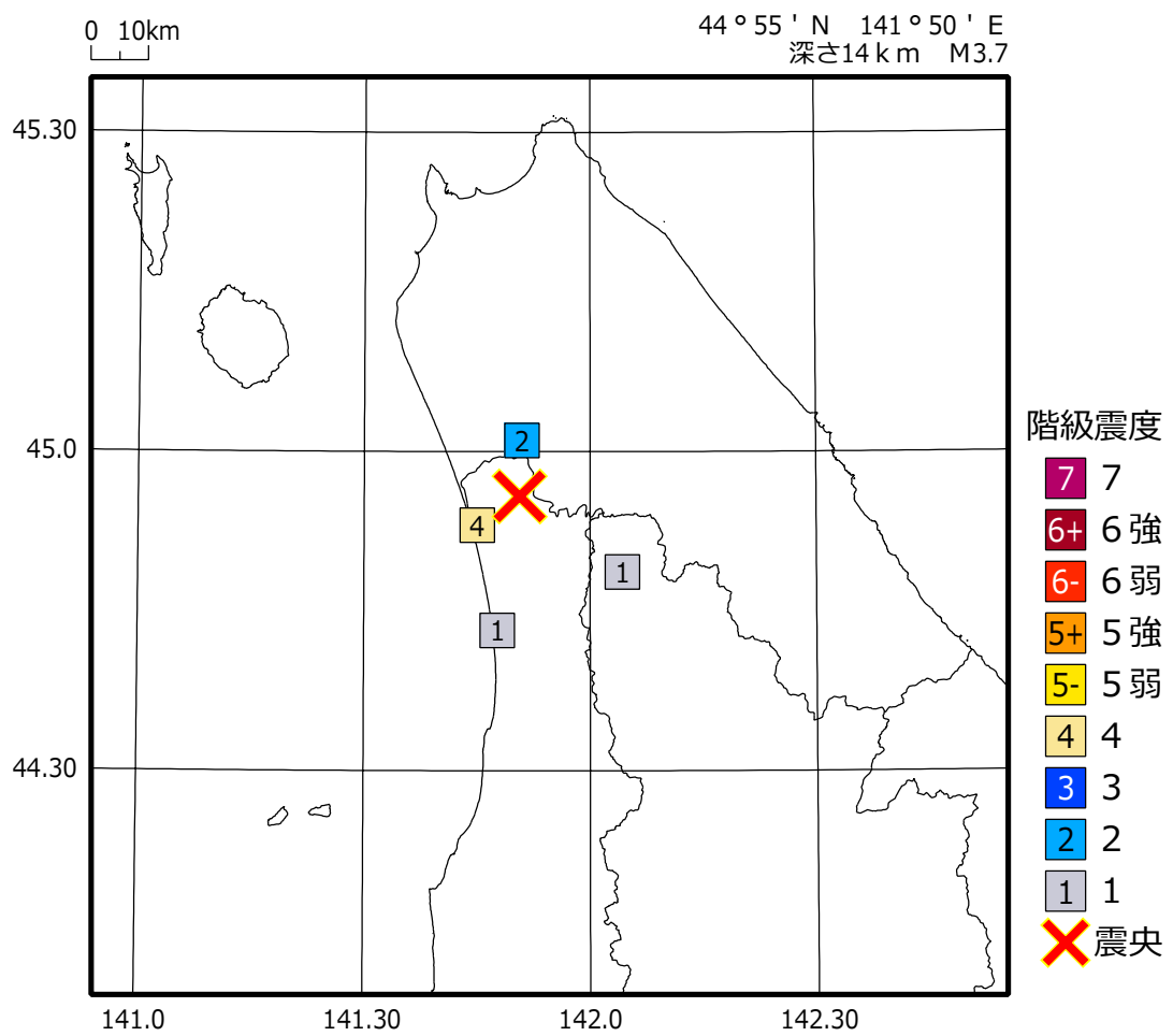
2024年 9月24日22時09分 留萌地方中北部の地震の震度分布図
