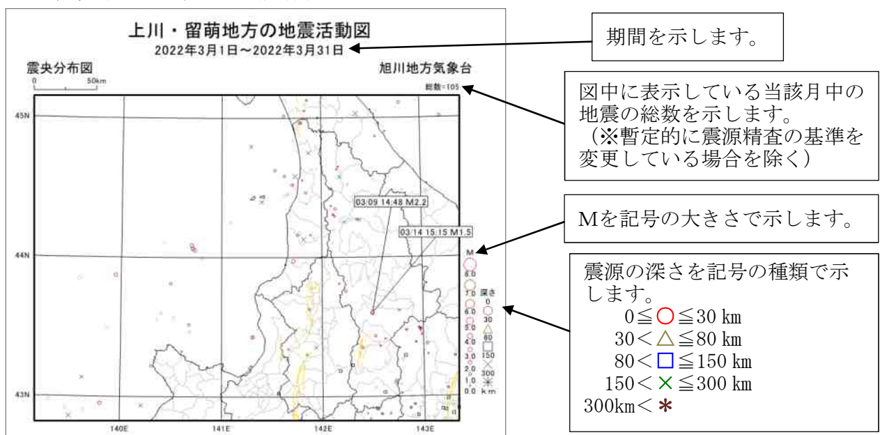
図1 震央分布図
