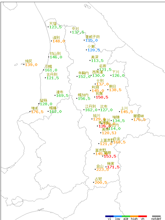
2024年10月 月降水量(mm)
