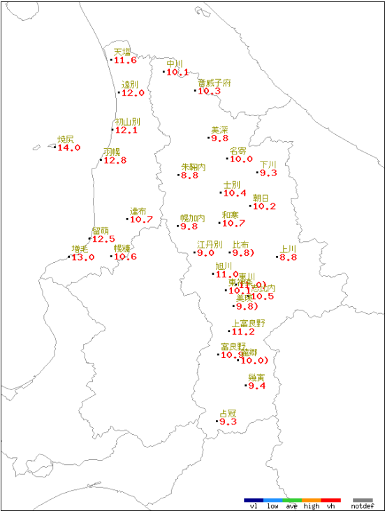
2024年10月 月平均気温(℃)
