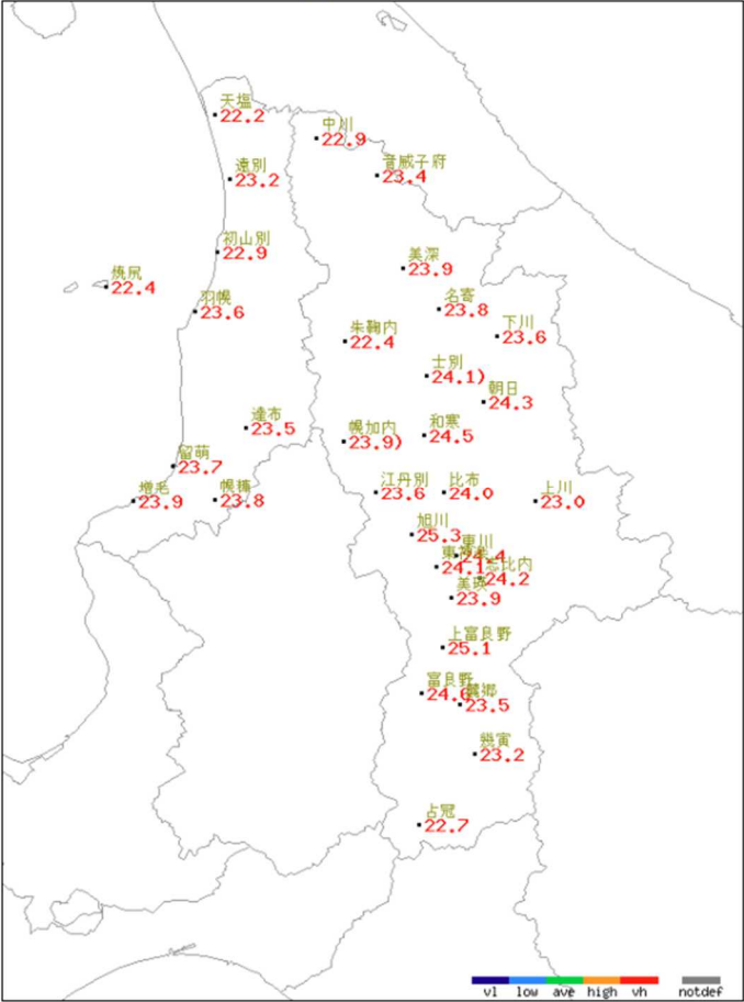
アメダス月別値 2025年7月 平均気温(℃)
