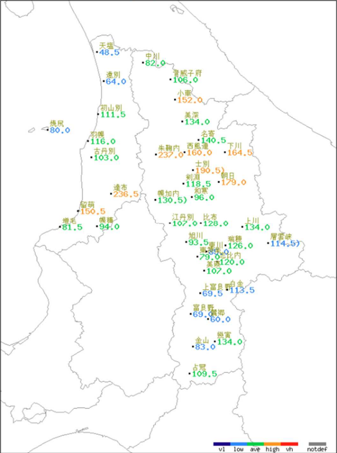
アメダス月別値 2025年7月 降水量(mm)
