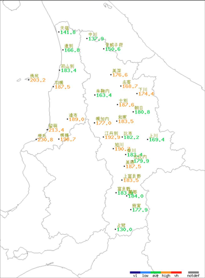
アメダス月別値 2025年7月 日照時間(h)
