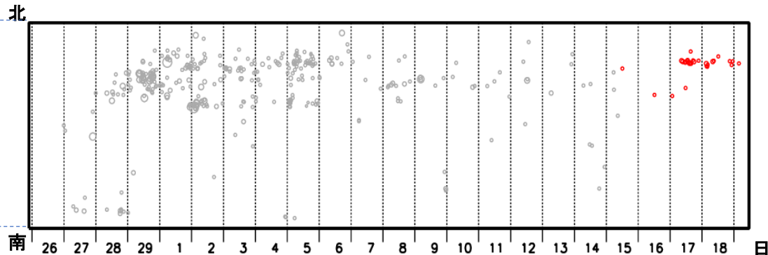
震央分布図の矩形内の時空間断面図
