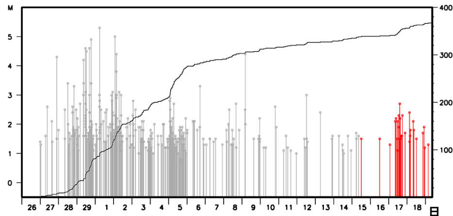
震央分布図の矩形内の地震活動経過・回数積算図
