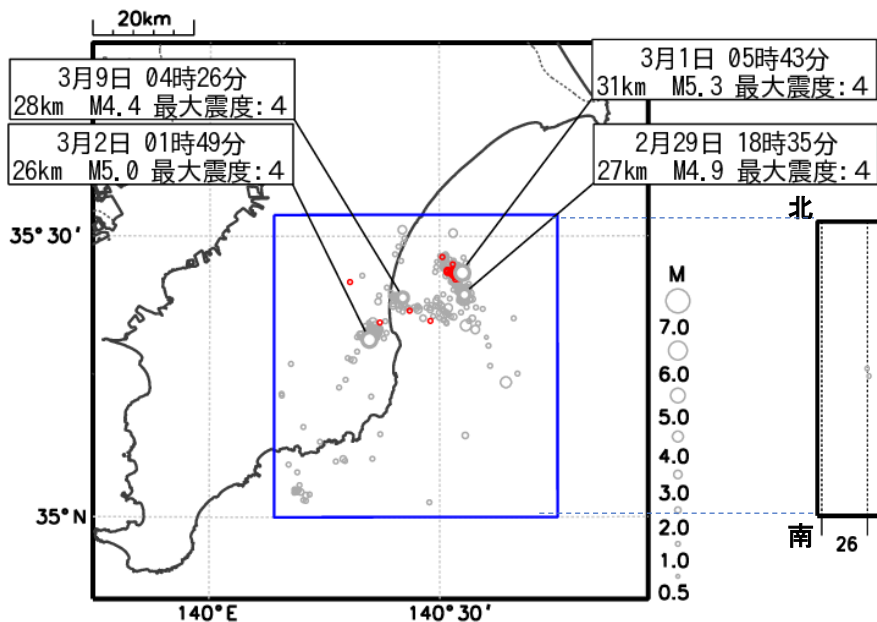
震央分布図
