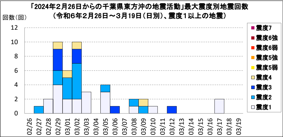
【最大震度別・日別地震回数グラフ】
